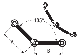
Grab Bar 135°
